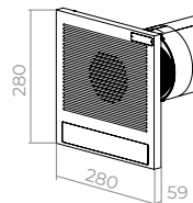
Climtec Quattro 150, 200+
