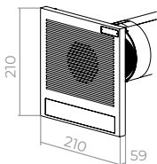
Climtec Quattro 100, 125
