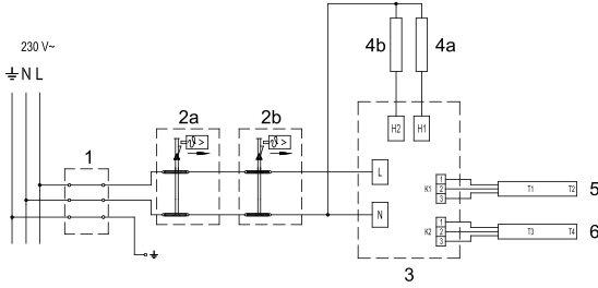
Рисунок 6: Электросхема
