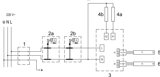
Мал. 6: Електросхема
