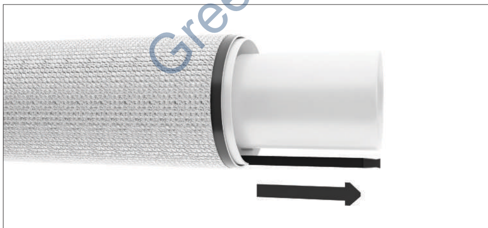
Зображення 2.8. Дотягування догрівуючого елемента на всю довжину внутрішнього хвостового каналу.
