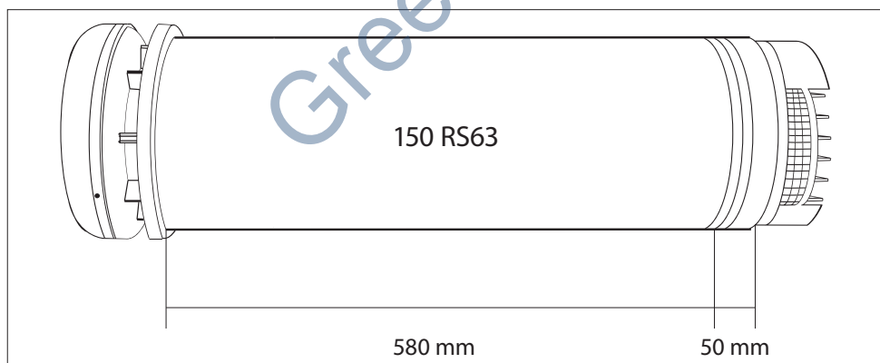
Зображення 1.5. Габаритні розміри рекуператора PRANA 150-ї серії у виконанні RS63.
