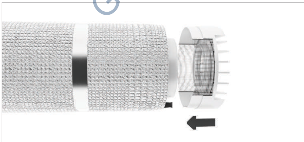
Зображення 2.12. Монтаж зовнішньої кришки рекуператора та місцерозташування отвору конденсатовідводу.
