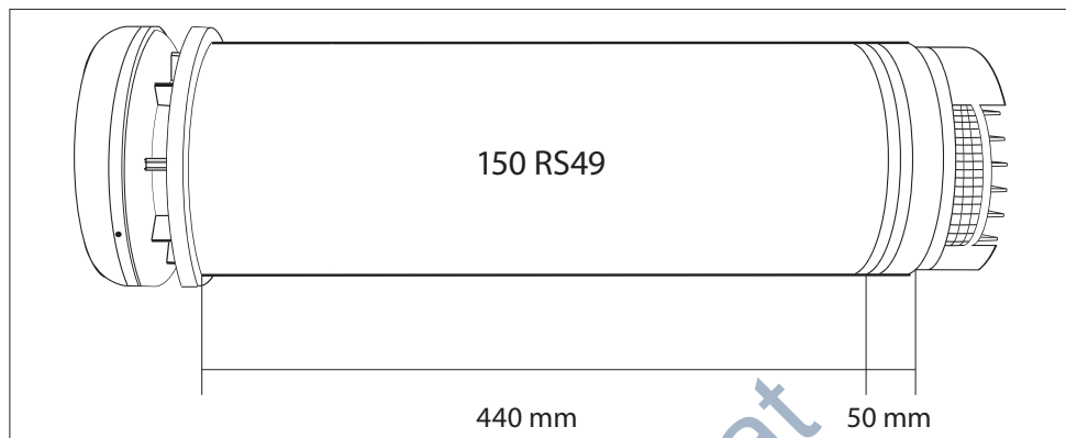
Зображення 1.4. Габаритні розміри рекуператора PRANA 150-ї серії у виконанні RS49.
